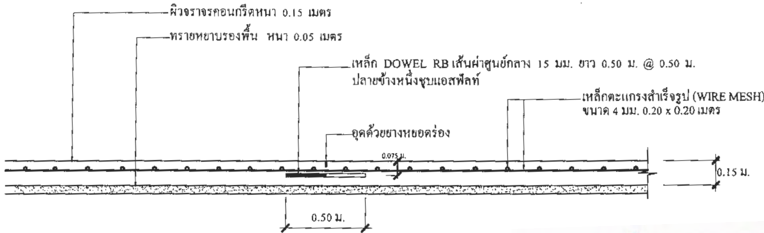
CONTRACTION JOINT ทุกระยะไม่เกิน 10.00 เมตร
