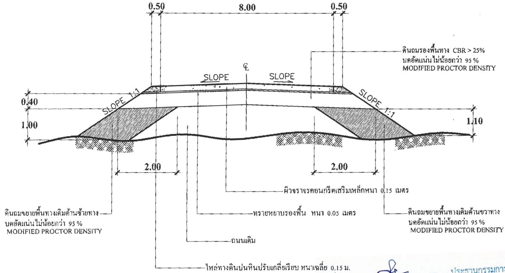
รูปตัดแสดงโครงสร้างถนน STA 1+300 ถึง 1+400
