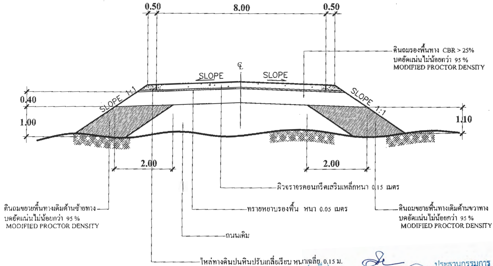
รูปตัดแสดงโครงสร้างถนน STA 1+400 - 1+500
