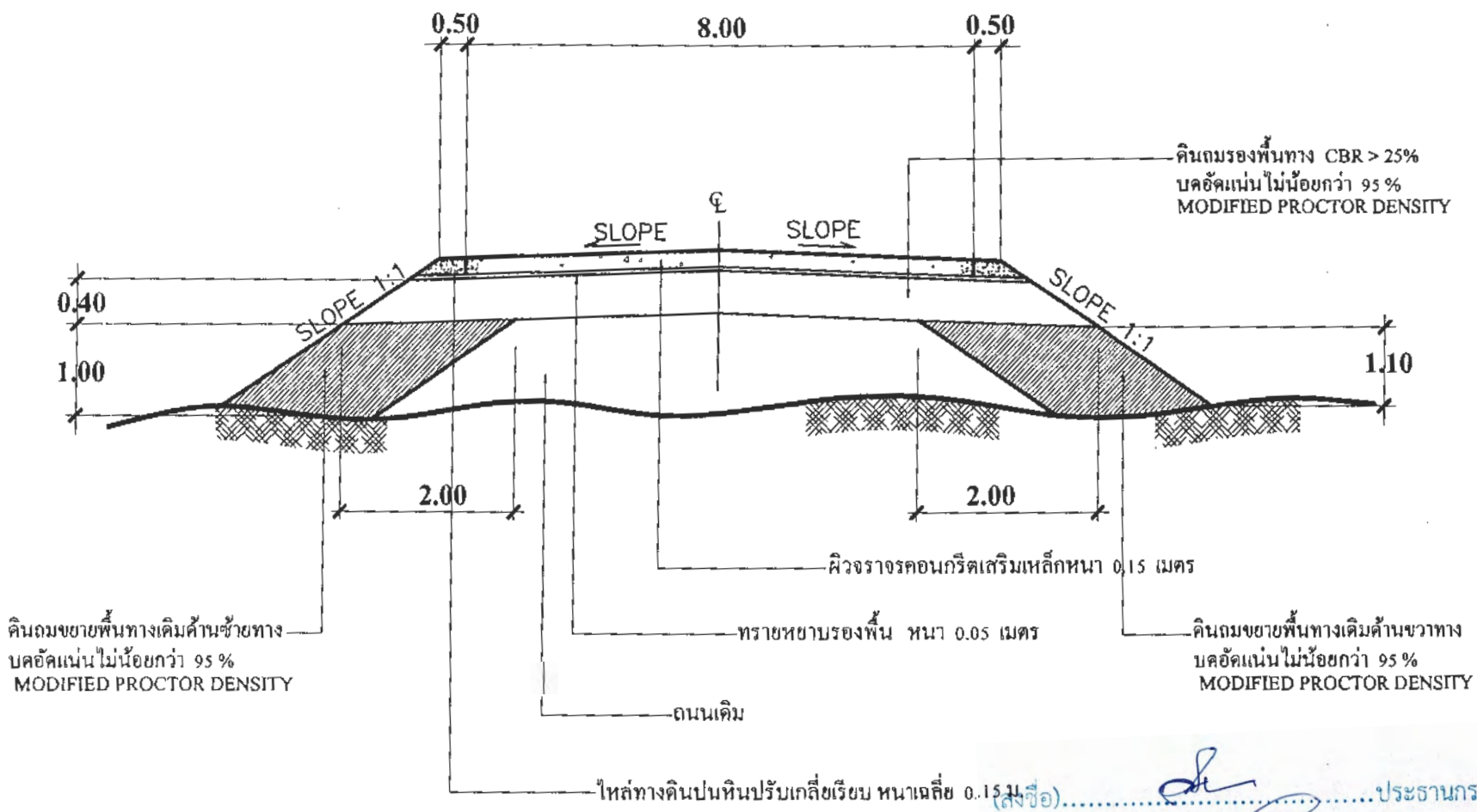
รูปตัดแสดงโครงสร้างถนน STA 0+900 - 1+000
